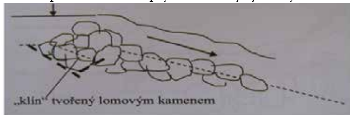
Obr. 22 Zpevňující klyn z balvanů (Šlezinger 2010)
